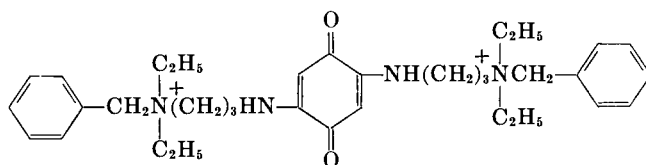
Mytolon (benzoquinonium)
