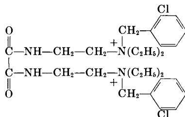
Ambenonium
