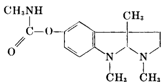
Eserine
