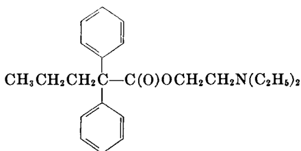
SKF 525A
